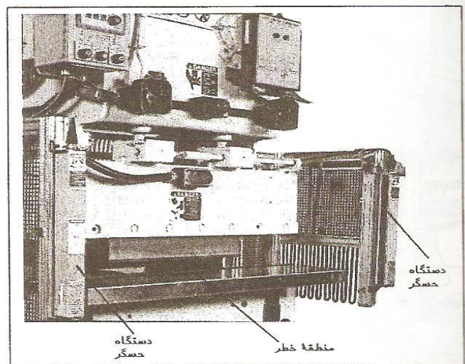
سیستم فتو الکتریک در پرس دارای کلاچ یا گیرش جزئی
